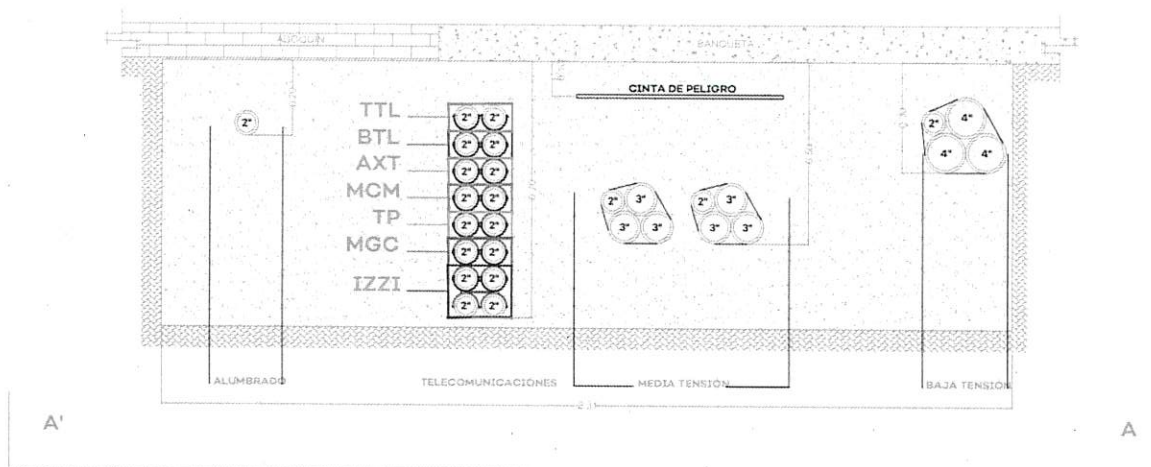
DETALLE CANALIZACION EN BANQUETA TUBERIA PAD RD-17
